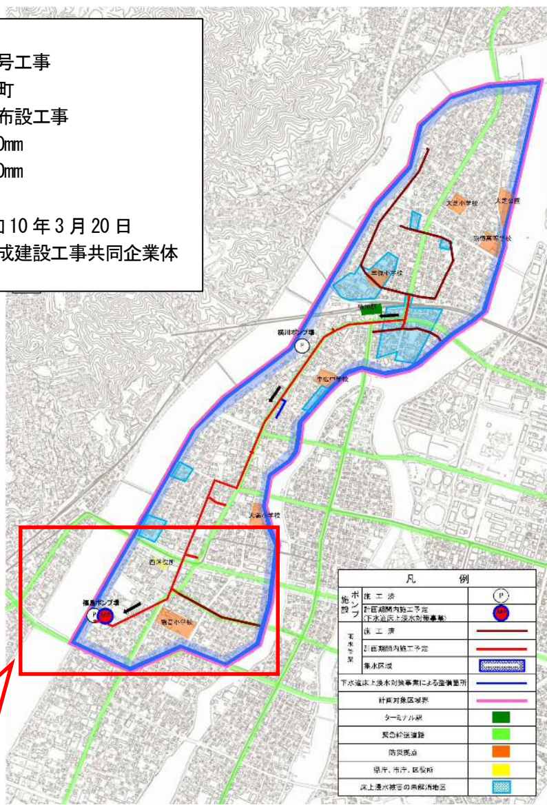
広島市三篠・観音地区大規模雨水処理施設整備事業概要図 (出典：広島市HPより)
